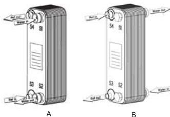
Figur 4. Installation som fordampere (A) og kondensator (B).
