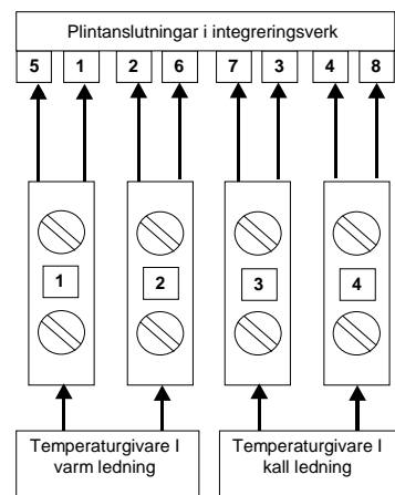
Fig. 5: Kabelanslutning, temperaturgivare
