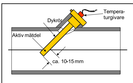
Fig.6: Exempel på montering för nominella storlekar \leq DN 40
