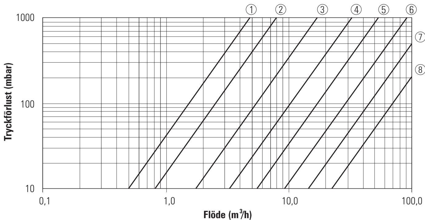
Tryckfallsdiagram
